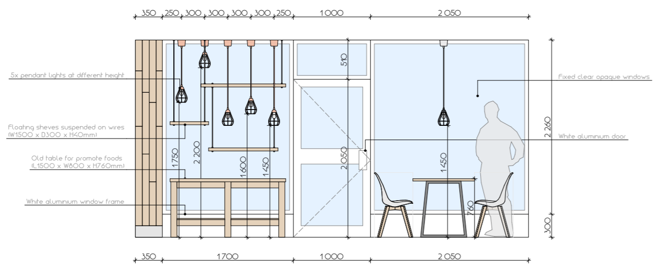
2 ELEVATION ENTRY WALL OPTION 01 A-2 SCALE: 1:50
