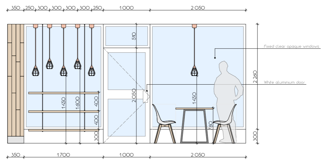
2 ELEVATION ENTRY WALL OPTION 02 A-2 SCALE: 1:50
